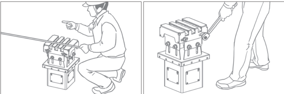
⑧⑥⑦で位置を確定させた中央部のベルベースから、長手方向両側へ順番にそれぞれ定められた間隔に合わせる。 ⑨頭部4本の高力ボルトを1次締めする (1次締めのトルク値は100N・mとする)。 1次締めした高力ボルトに黒または白の油性マーカーを用いてマーキングをする。
