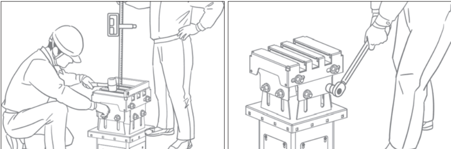
③他のベルベースの頭部を基準レベルに合わせて水平に調整する。 ④連結部の8本の高力ボルトを1次締めする (1次締めのトルク値は100N・mとする)。
