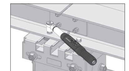
⑥ボルト頭を所定のトルク値で締め、抜け止めバーをセットする。
