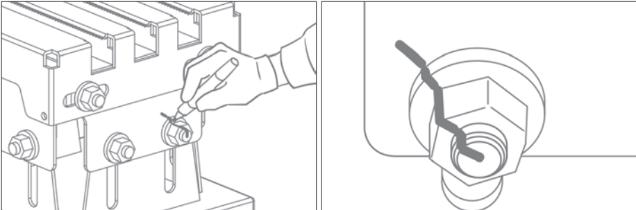
⑤1次締めした高力ボルトに黒または白の油性マーカーを用いてマーキングをする。 マーキングの方法
