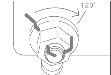
本締めは、1次締付け完了後を起点とし て、ナットを120°回転させて行なう。
