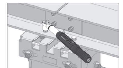
⑥ボルト頭を所定のトルク値で締付、 抜け止めバーをセットする。
