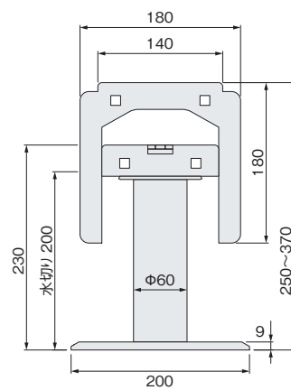
正面図 VBKA H250
